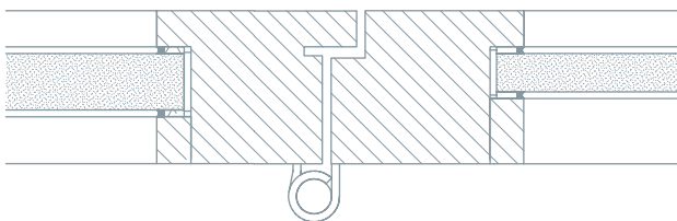
Anschluss Cristallo-Tür EI30 ans freie Glasumfeld EI60
