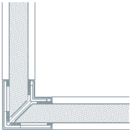
Eckstoß 90° Cristallo-Wand EI30 / EI60 mit thermostabilem Jegen Spezialeckprofil (Patent-Nr. EP 2746519B1)
