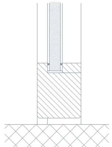
Bodenanschluss Cristallo-Tür EI30
