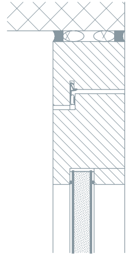
Cristallo-Tür EI30
