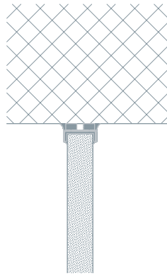
Deckenanschlussprofil Typ 1 Cristallo Wand EI30 / EI60
