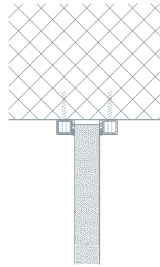
Deckenanschlussprofil Typ 2 Cristallo Wand EI30 / EI60
