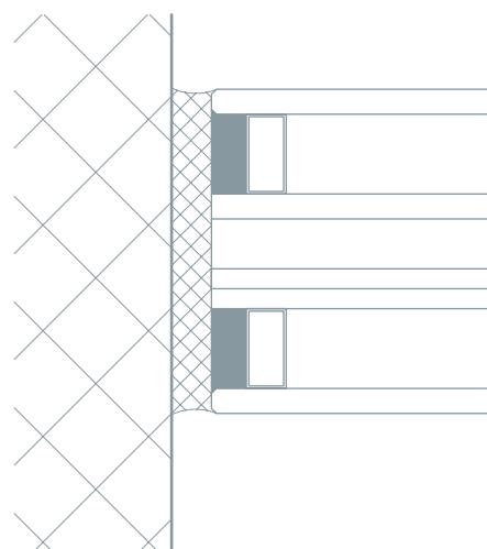
Wandanschluss Festfeld EI60
