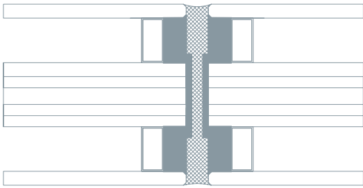
Glasstoss Festfeld EI60
