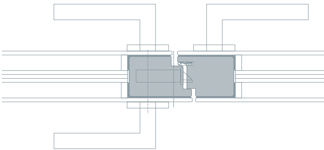
Mittelpartie EI30 (2-flg.)
