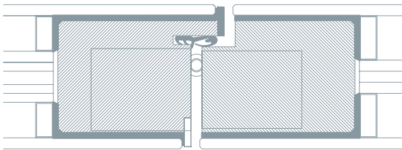
Anschluss Bandseite EI30 an Festfeld EI60
