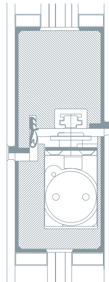
Türflügel EI30 oben
