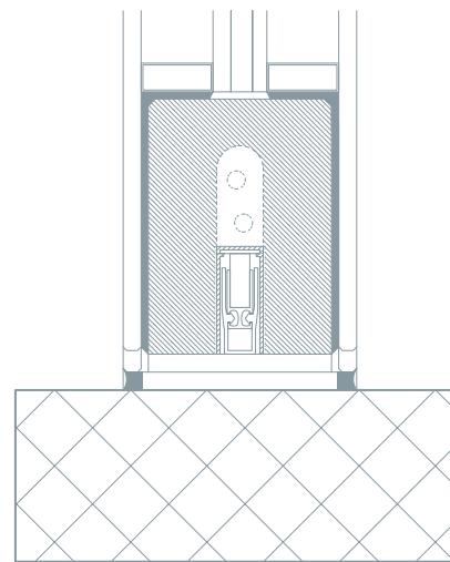
Türflügel EI30 unten
