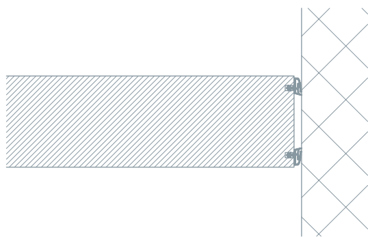
Horizontalschnitt Wandanschluss
