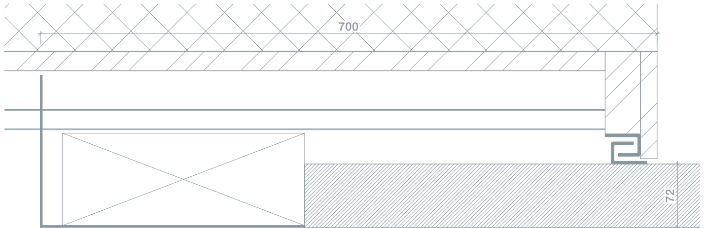
Horizontalschnitt Antriebsseite
