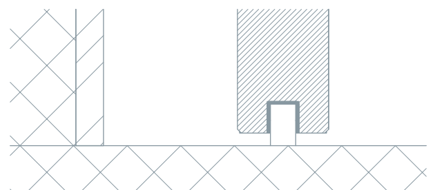
Vertikalschnitt Bodenanschluss
