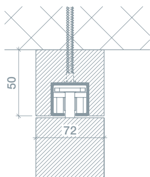
Wandnische
