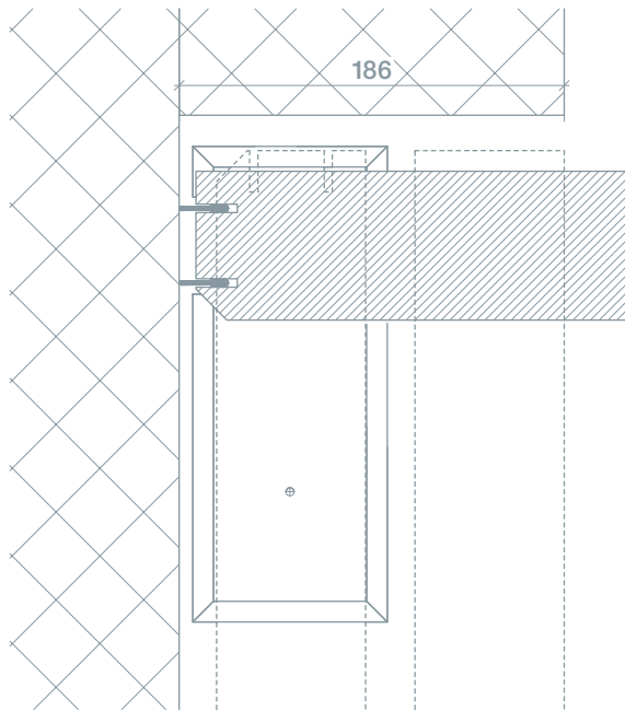
Flügelmittelpartie
