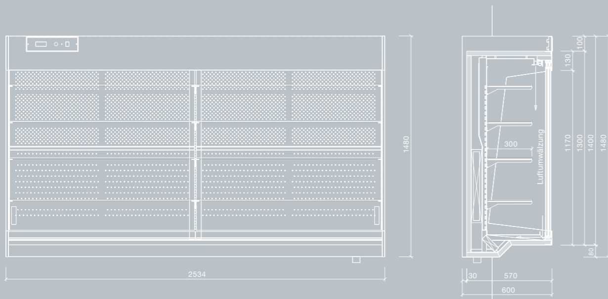
Ansicht
