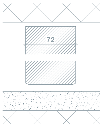
Deckenanschluss 1 Rahmenlos unter Decke
